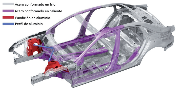
Estructura de carrocería.
