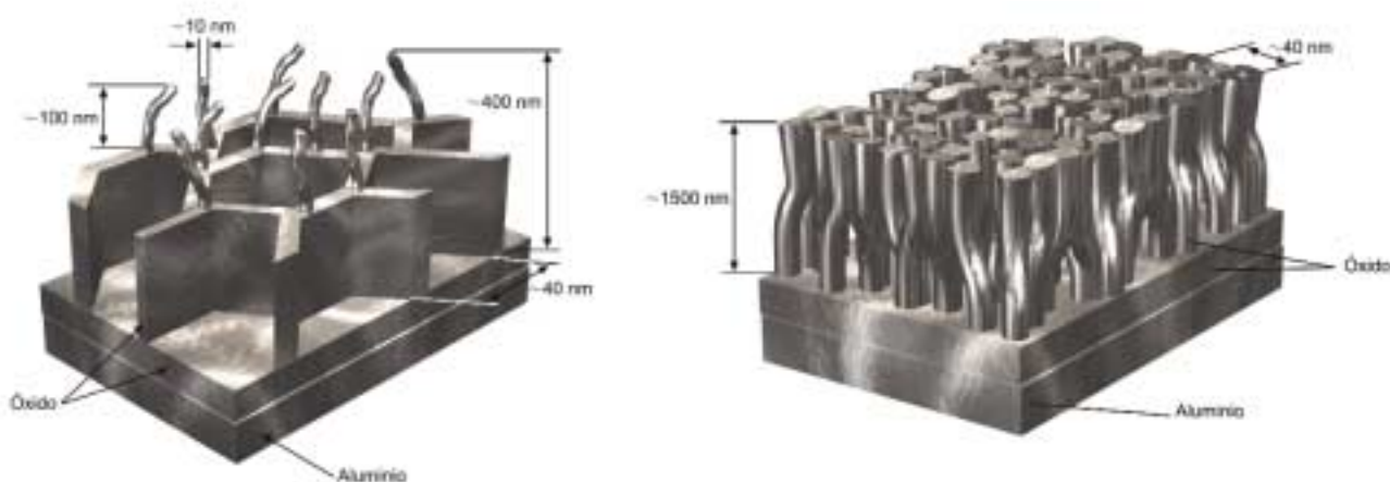
Figura 2.- Geometrías de los óxidos producidos por diferentes técnicas de ataque químico sobre un sustrato de aluminio. El espesor es del orden de una micra.
